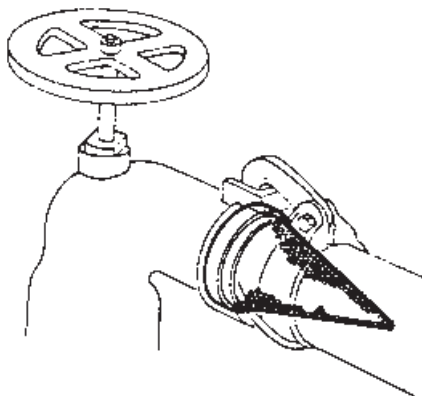
شکل ۱۶-۹- ورق صافی که در ابتدای لوله جانبی مورد استفاده قرار می گیرد.
