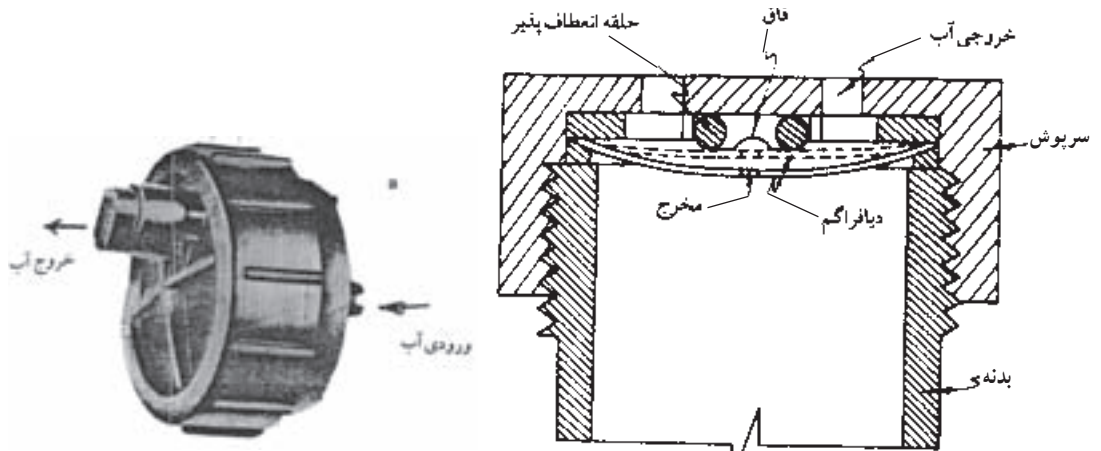
د) قطره چکان دارای دیافراگم
