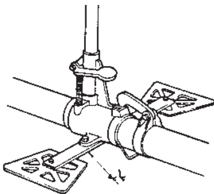
شکل ۱۷-۹- پایه آبیاش
