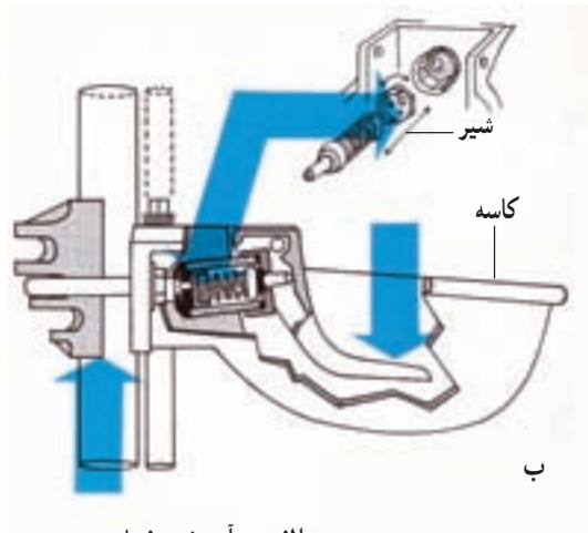
الف - آبشخور فشاری
