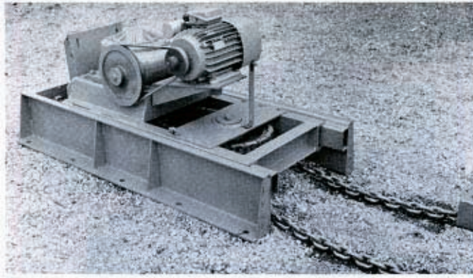
شکل ۲۶-۴- الکتروموتور و زنجیر محرک تیغه
