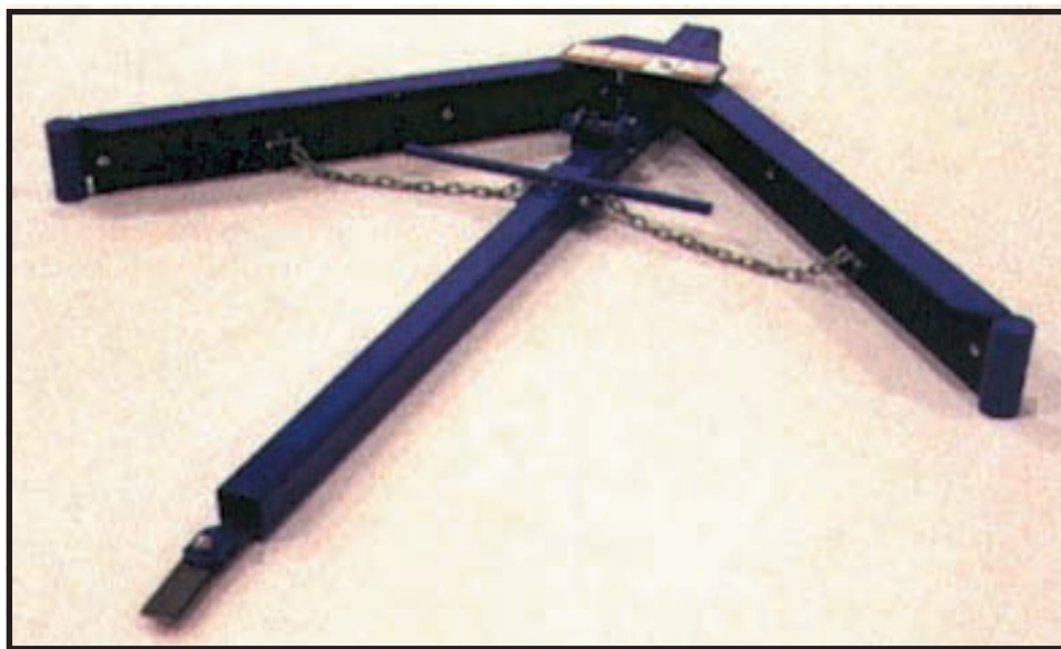
شکل ۲۵-۴- تیغه جمع‌آوری فضولات
