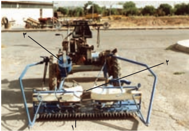
۱- شانه برش ۲- دهانه دسته‌بند ۳- محافظه محتوی دوک نخ شکل ۸- ۸- واحد درو دسته‌بند و اجزای آن
