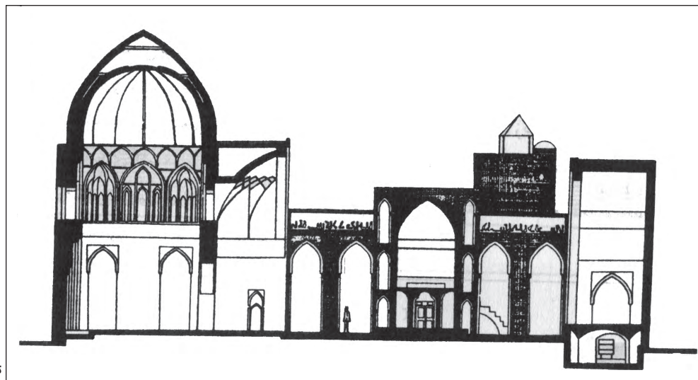
تصویر ۲۰-۵- سقف دو پوسته در گنبد
