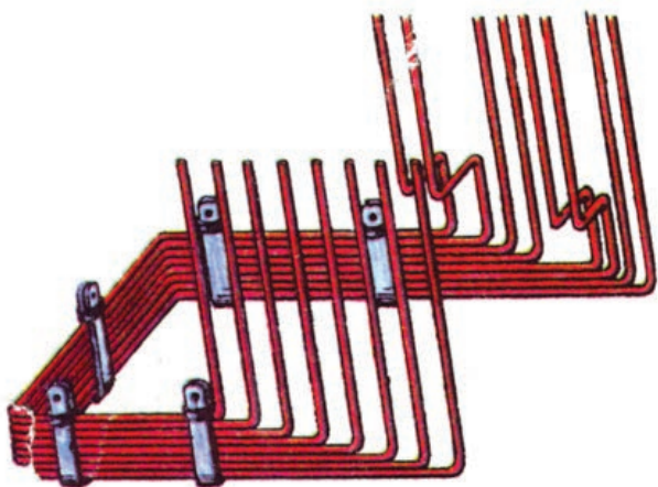
شکل ۳-۹- فرم‌کاری سیم‌ها
