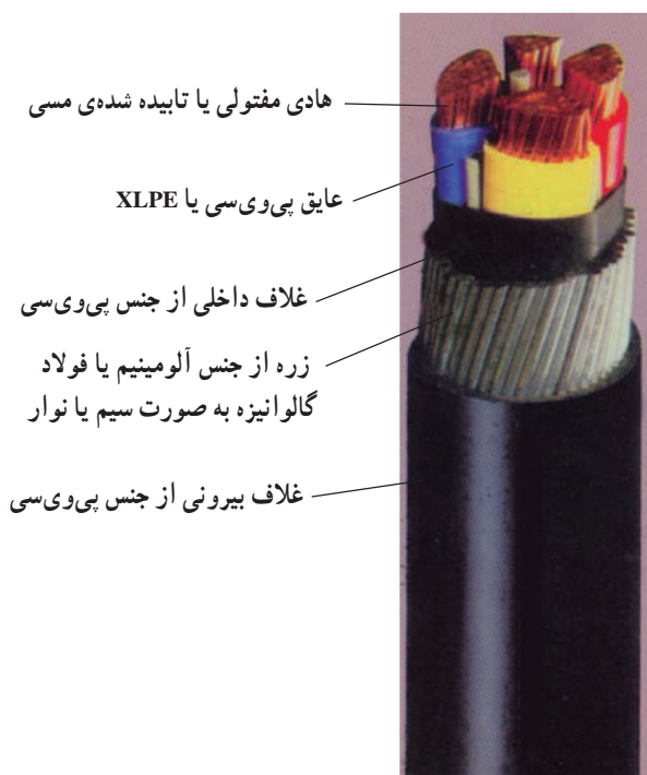
شکل ۴-۵- کابل با عایق PVC به همراه اجزای کابل
