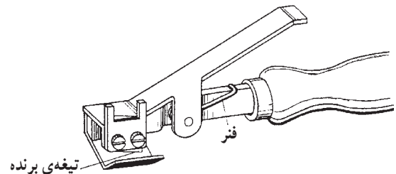
شکل ۵-۲۴- شیپار در آر طولی کابل
