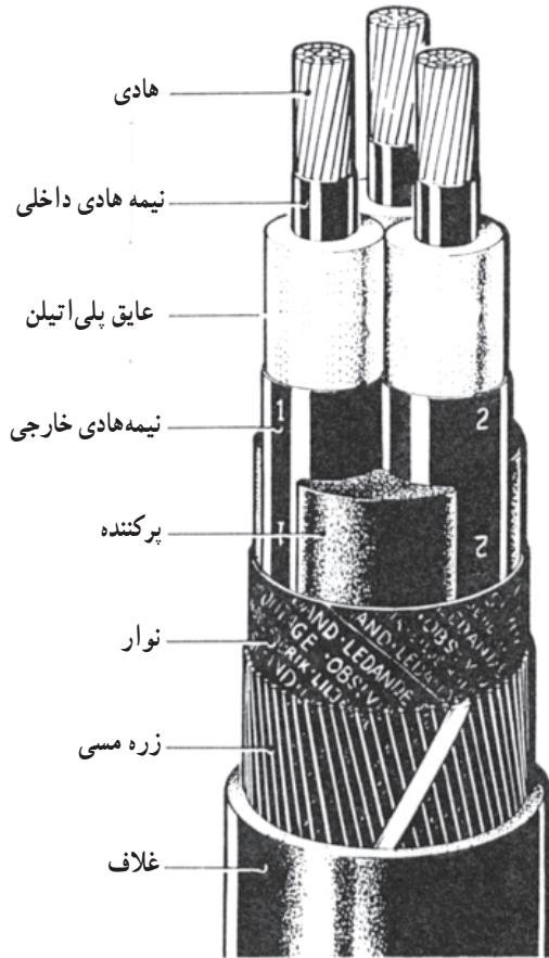
شکل ۵-۱-۵-۱- قسمت های مختلف یک کابل ۲۰ kV
