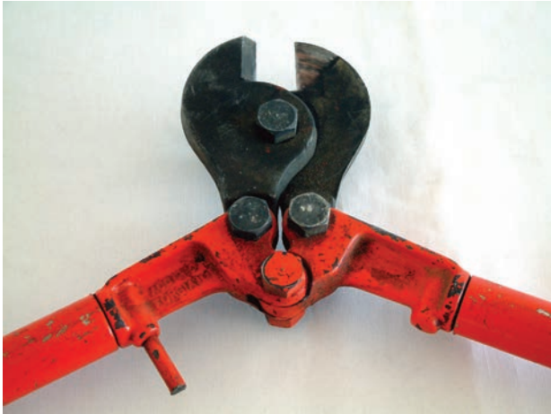
شکل ۵-۷۳- قیچی کابل‌بری
