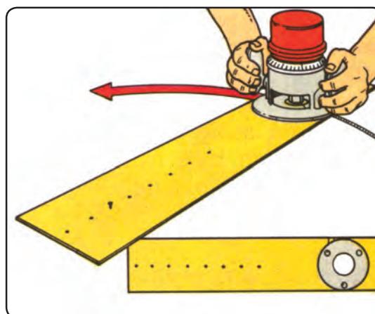
شکل ۵۴-۲ فرزکاری با شابلون دایره
