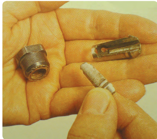
شکل ۲-۴۱ بوش تیغه اور فرز همراه با مهره سفت‌کننده تیغه روی شفت دستگاه
