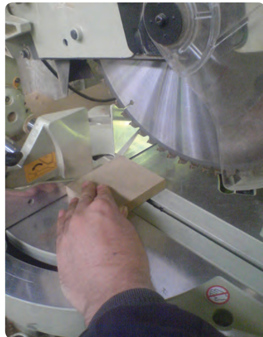
شکل ۲-۱۶ - عدم رعایت نکات ایمنی برای برش قطعات کوچک‌تر
