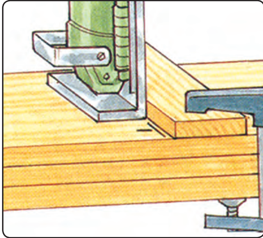
شکل ۸۶-۲ اتصال زنی به کمک قطعه چوب گونیایی
