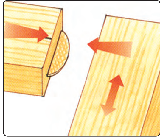
شکل ۸۴-۲ نحوه جازدن اتصال بیسکویتی
