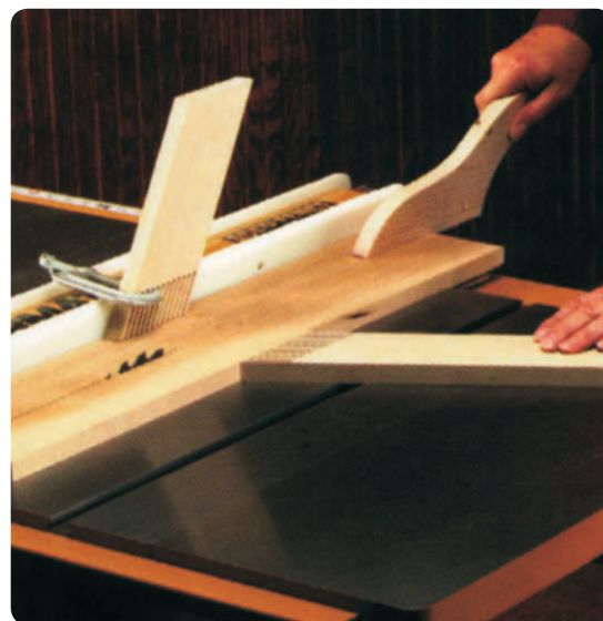
شکل ۳-۱۵ شابلون‌های حفاظتی در اره گرد
