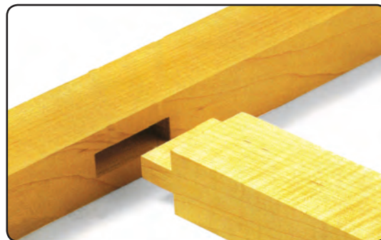
شکل ۳۶-۴ اتصال کُم و زبانه مخفی (یک طرفه)
