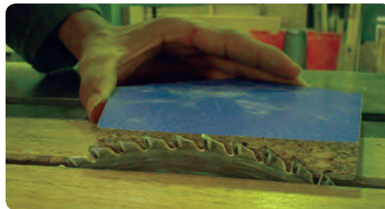
شکل ۳-۳۸ تنظیم ارتفاع تیغه اره
