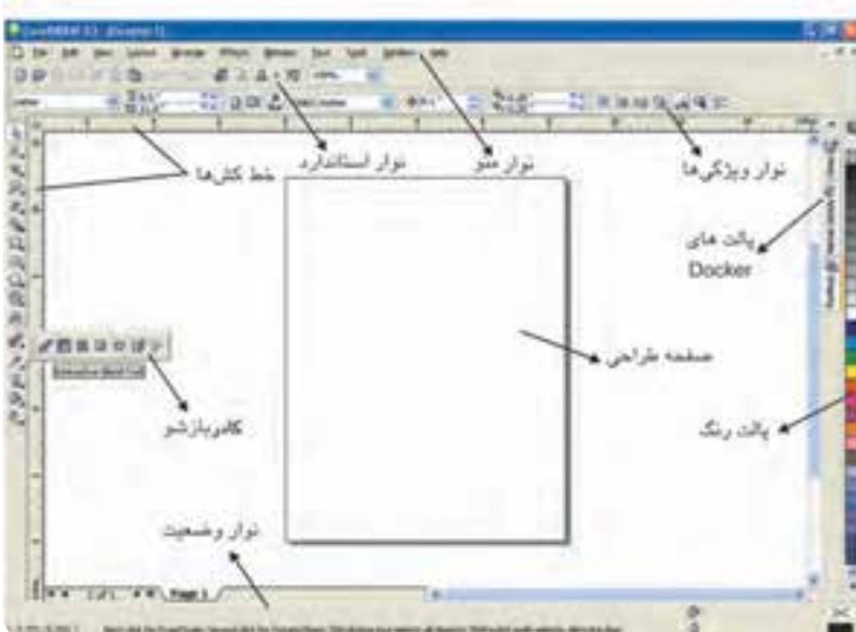
شکل ۲-۱ پنجره CorelDRAW
