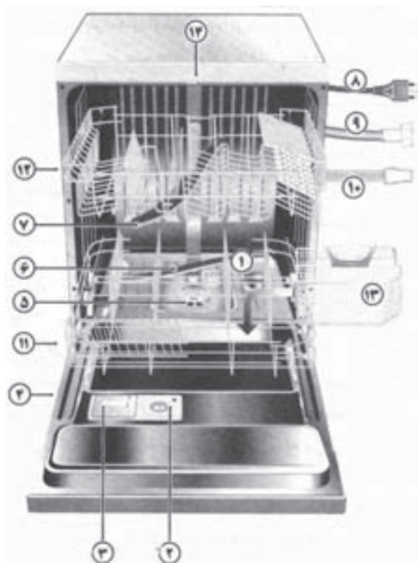
شکل ۱۶-۶- اجزای ماشین ظرفشویی اتوماتیک
