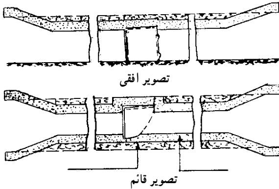
شکل ۲-۳۹- مقاطع دیافراگم
