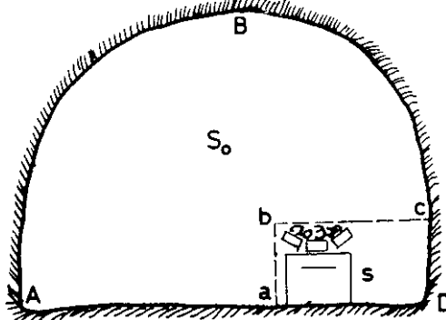
شکل ۱۱-۲- اثر تجهیزات ثابت در کم شدن سطح مقطع عبور هوا
