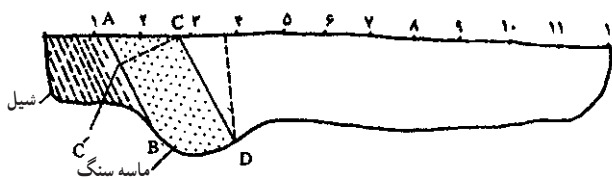
شکل ۱۴-۱۰- برداشت لایه‌ها با تعیین دو نقطه بالا و پائین آنها در ترانسه [۲۳]
