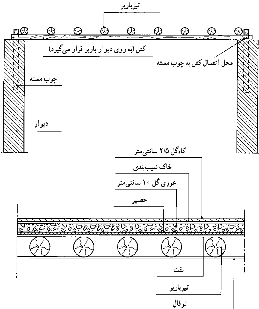
شکل ۲- مقاطع سقف تخت چوبی
