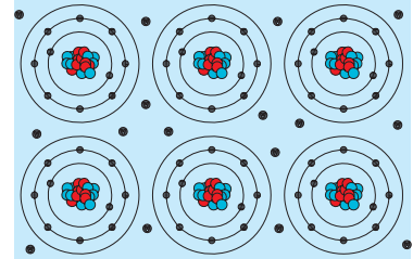
شکل ۱-۲۷ دریای الکترونی در پیوند فلزی
