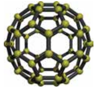
شکل ۶-۶ مولکول C60
