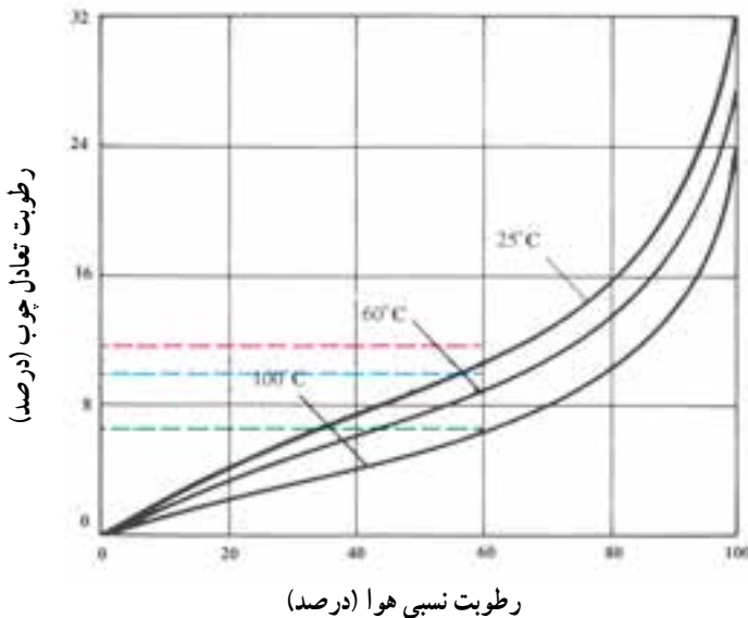
شکل ۱۲-۱ – منحنی تغییرات رطوبت چوب در شرایط رطوبت نسبی و درجه حرارت متفاوت
