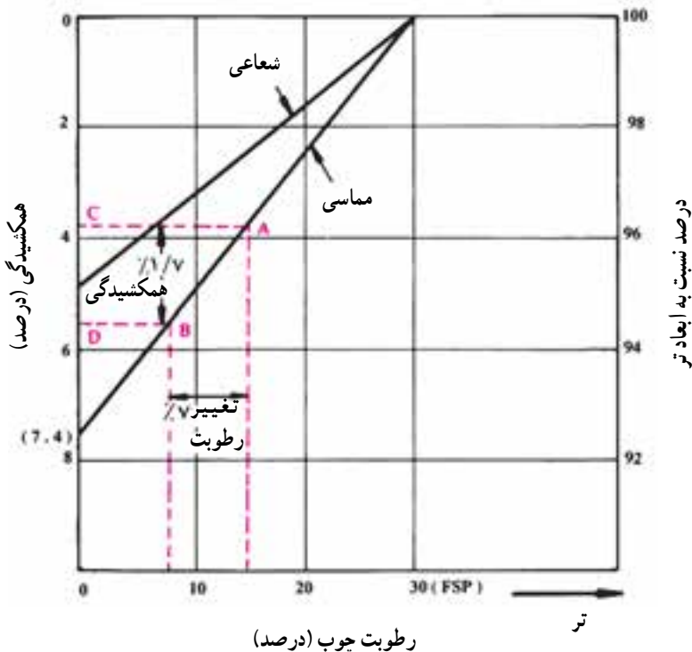
شکل ۱-۲۷- برآورد همکشیدگی و تغییر ابعاد چوب در اثر دفع رطوبت
