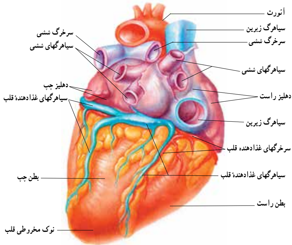
شکل ۱۲-۷- تشریح قلب
