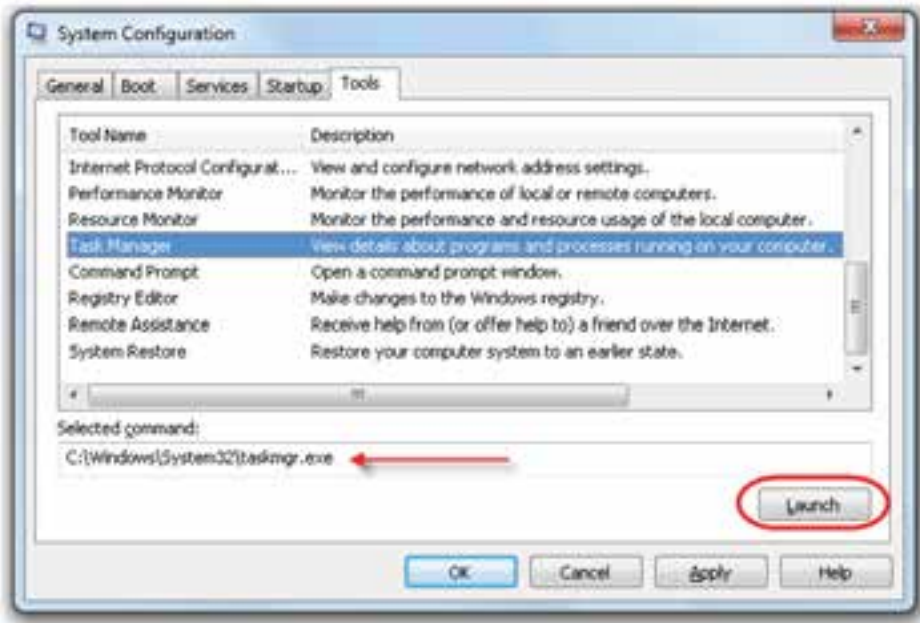
شکل ۱۴-۳۔ زبانہی Tools از برنامہی System Configuration
