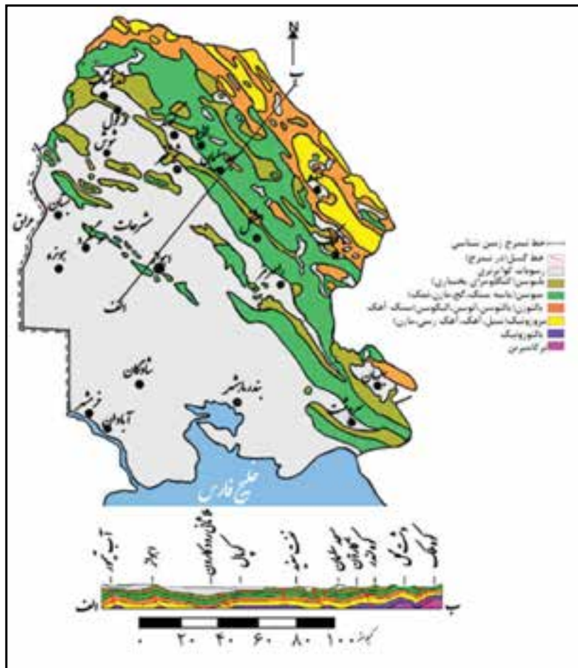
شکل ۸-۱- نیمرخ زمین‌شناسی استان
