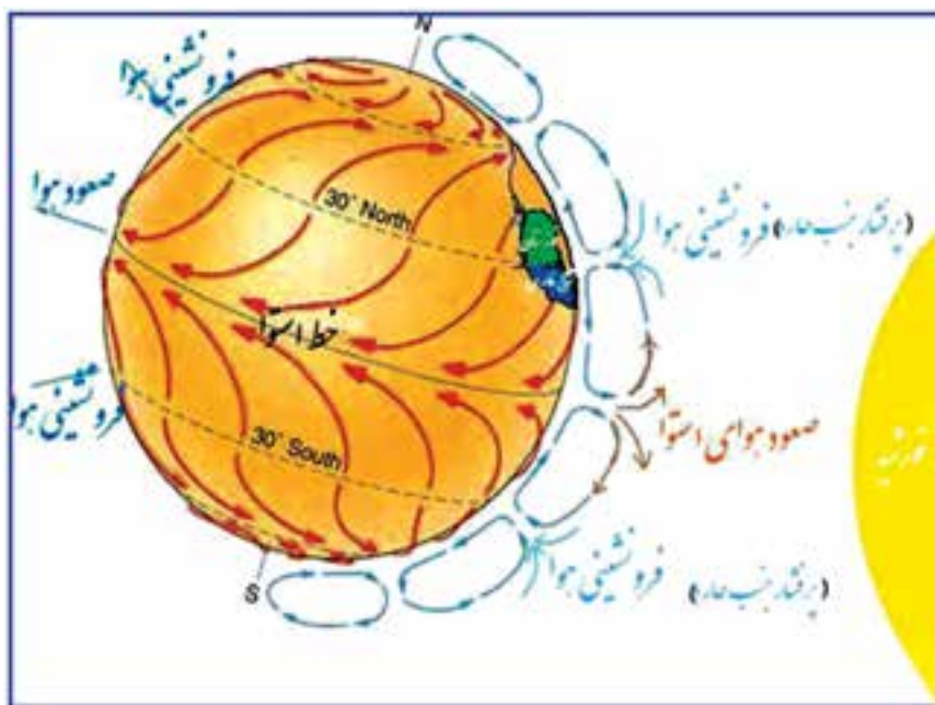
شکل ۱۳-۱- تأثیر پرفشار جنب حاره بر آب و هوای استان
