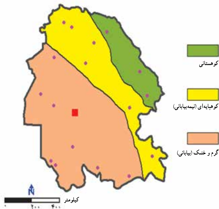
شکل ۱۷-۱- انواع مناطق آب و هوایی استان
