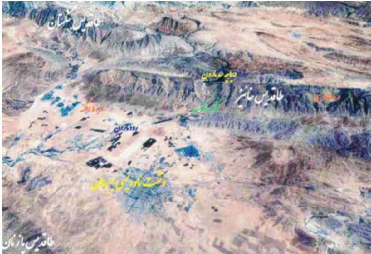
شکل ۱۰-۱- تصویر ماهواره‌ای از ناقدیس‌های جنوب شرق استان
