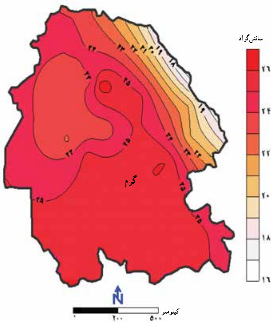
شکل ۱۴-۱- نقشه هم دمای سالانه استان
