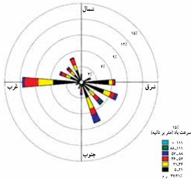
شکل ۱۶-۱- گلباد ایستگاه هواشناسی اهواز
