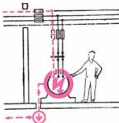
شکل ۲-۳ خط‌های اتصال بدنه، اتصال کوتاه و اتصال زمین
