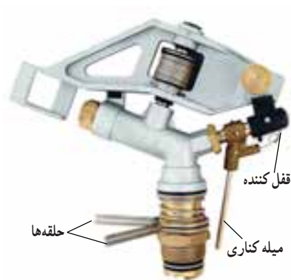
شکل ۲۱-۷- ساختمان آب پاش سکتوریل
