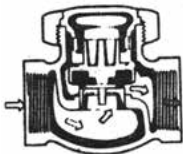
▲ شکل ۸-۷- قسمت‌های مختلف یک شیر یک طرفه سوپابی
