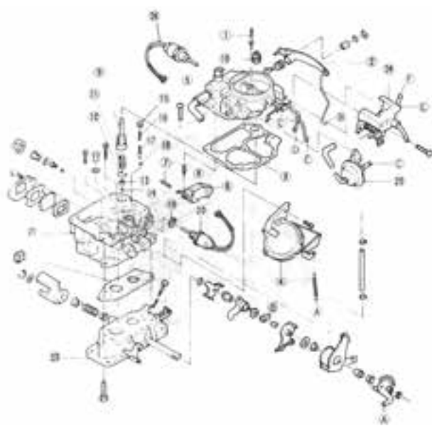
شکل ۱-۱۱۶ ترتیب باز کردن قطعات کاربراتور
