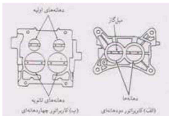
شکل ۱-۶۵ کاربراتورها از نظر دهانه
