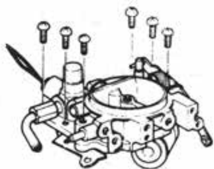
شکل ۱-۱۱۷ دهانه بالای کاربراتور
