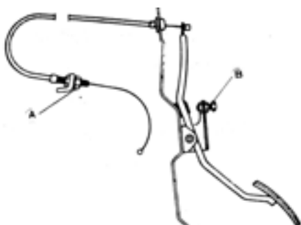
شکل ۱۲۱- ۱ سیم گاز و اتصالات A و B قابل تنظیم
