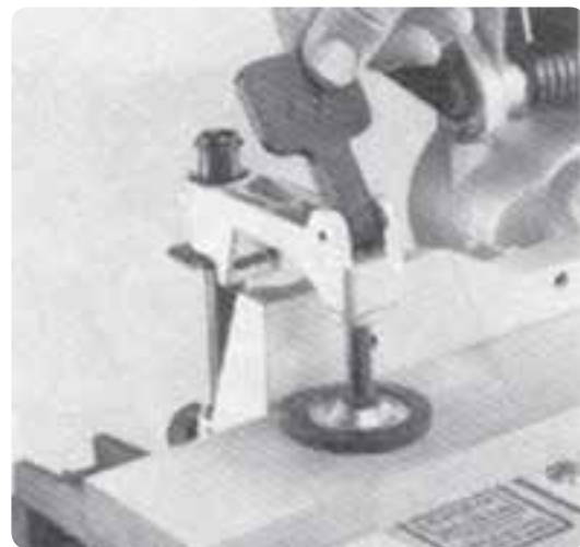
شکل ۲-۱۱- بستن قطعه کار با گیره
