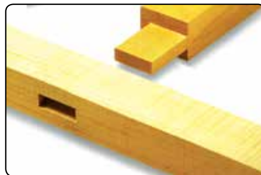
شکل ۳۷-۴ اتصال کُم و زبانه ساده (دو طرفه)
