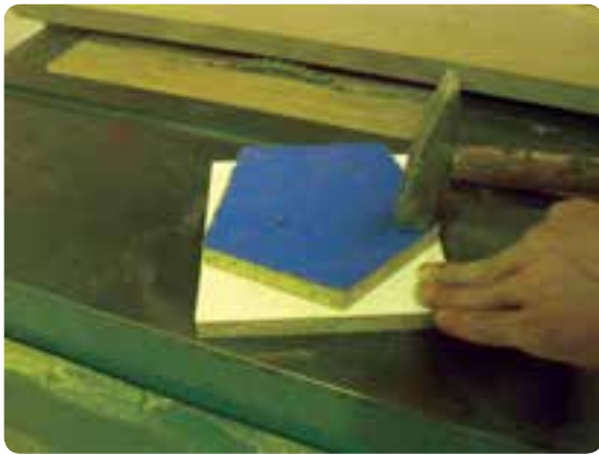
شکل ۳۷- ثابت کردن شابلون روی صفحه
