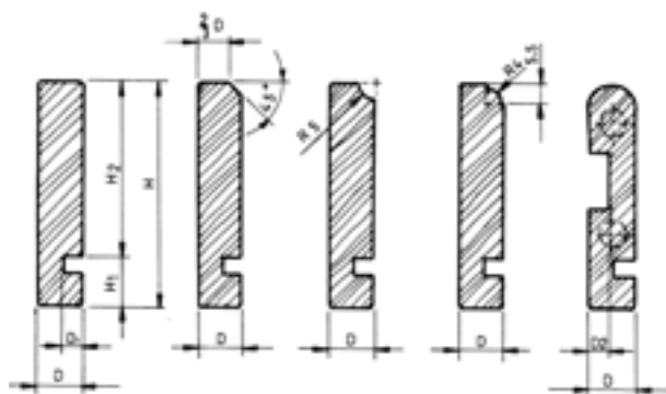
شکل ۶-۴۷ مشخصات انواع بدنه جعبه از چوب توپیر
