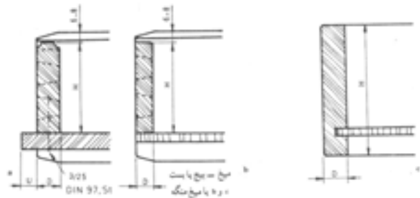
شکل ۶-۴۸ انواع عقب جعبه در برش عمودی
