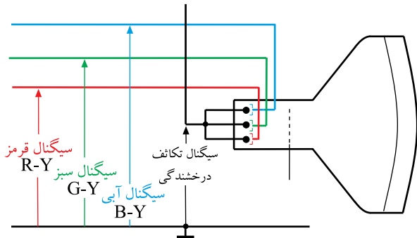
شکل ۱۰-۱- اتصال سیگنال‌های R-Y و B-Y و G-Y به شبکه
