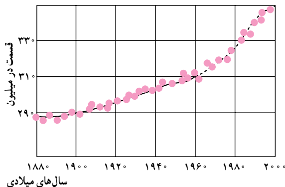
نوسان میزان دی‌اکسیدکربن هوا در دو قرن اخیر
