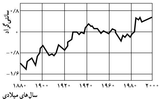
نوسان میزان دمای هوا در دو قرن اخیر
