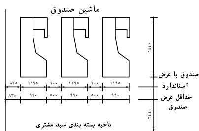
ابعاد و نقشه آرایش صندوق‌های پرداخت
