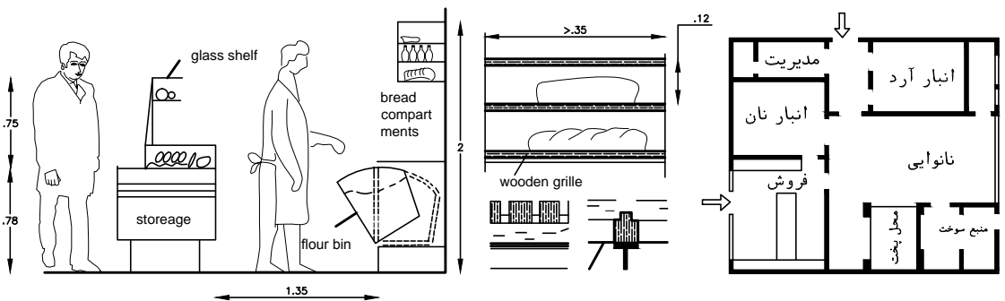
تصویر ۱۰-۵- سیر کولاسیون برای یک نانوایی تهویه دار
