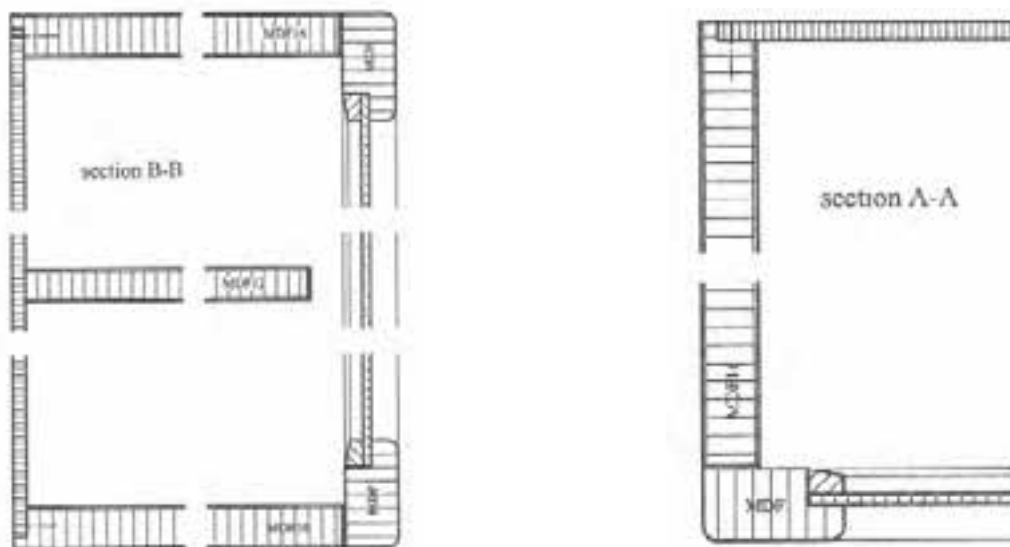
شکل ۱۲۸۳- نماها و برش‌های جمع‌بندی کمک‌های اولیه چوبی.
