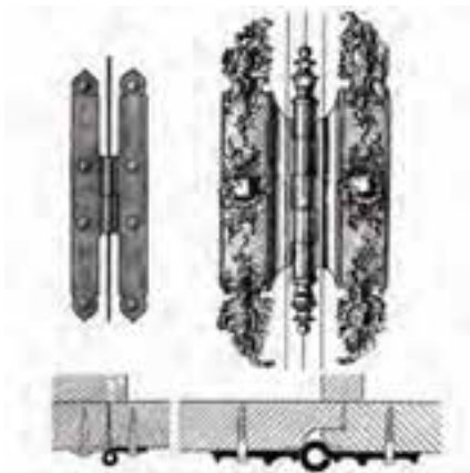
شکل ۱۰-۲۲- یک نوع لولای پروانه‌ای تزئینی؛ با مقطع نصب شده.
