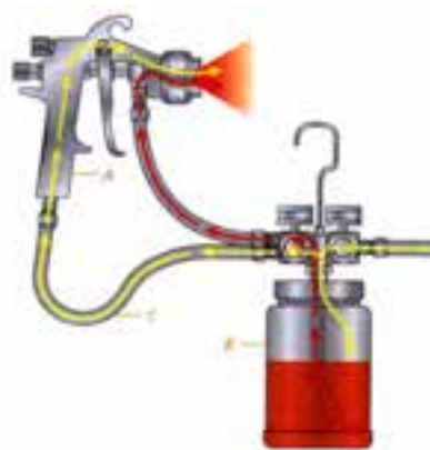
شکل ۳۴-۴- پیستوله با مخم کم.
