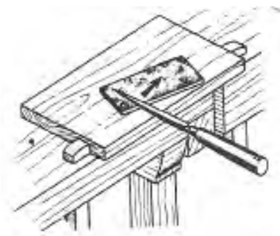
شکل ۲-۱۰- مصقل زدن لیسسه تا زاویه‌ی ۱۵ درجه.
