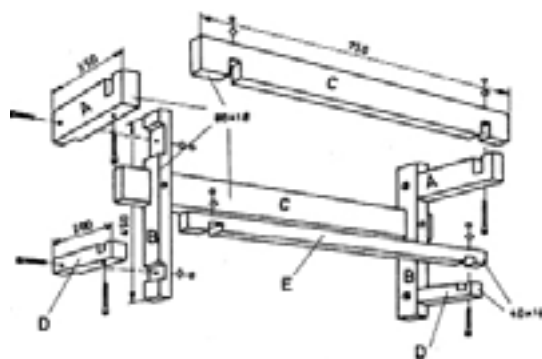
شکل ۹-۱۱۱- پرسبکتیو انفجاری آویز لوازم آشپزخانه.
