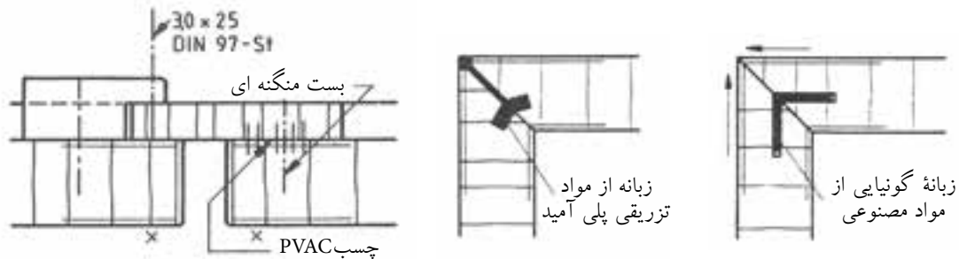
شکل (۴-۶۳) ترسیم علائم اتصال قلیف زبانه‌ی سراسری از جنس مواد مصنوعی شکل (۴-۶۴) ترسیم علائم اتصال قلیف سراسری تزریقی از مواد پلی‌آمید شکل (۴-۶۵) ترسیم علائم درز چسب با چسب PVAC و بست منگنه و پیچ فولادی
