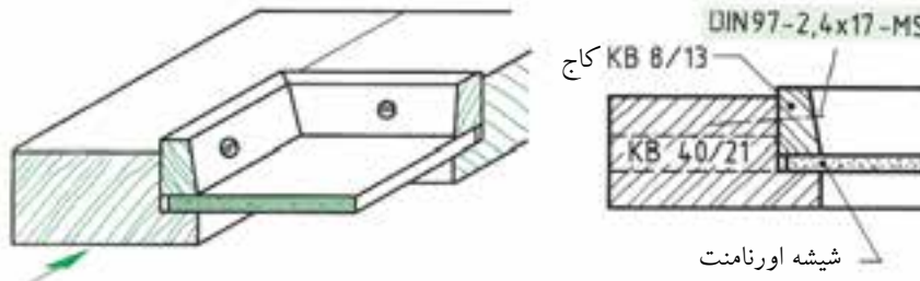
شکل (۴-۴۴) رسم علائم شیشه در برش پیشانی گوشه قاب و تصویر مجسم علامت KB = نوعی چوب کاج است.
