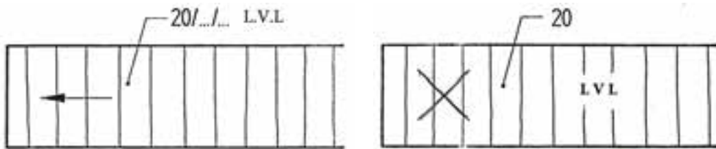
شکل (۴-۲۴) تخته L.V.L با ضخامت ۲۰ میلی متر با علامت راه چوب
