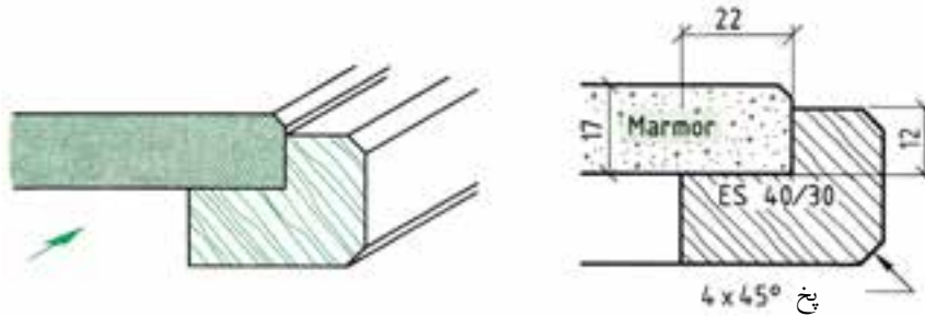
شکل (۴-۴۳) رسم علائم سنگ مرمر روی قاب و شیشه
