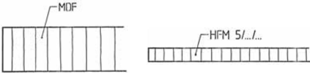
شکل (۴-۲۱) تخته فیبر نیمه سخت HFM با ضخامت ۵ میلی متر شکل (۴-۲۲) ترسیم نقشه تخته فیبر با دانسیته متوسط MDF
