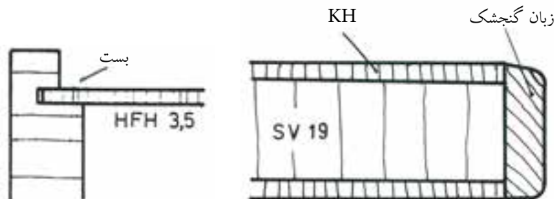
شکل (۴-۴۱) کاربرد HFH
