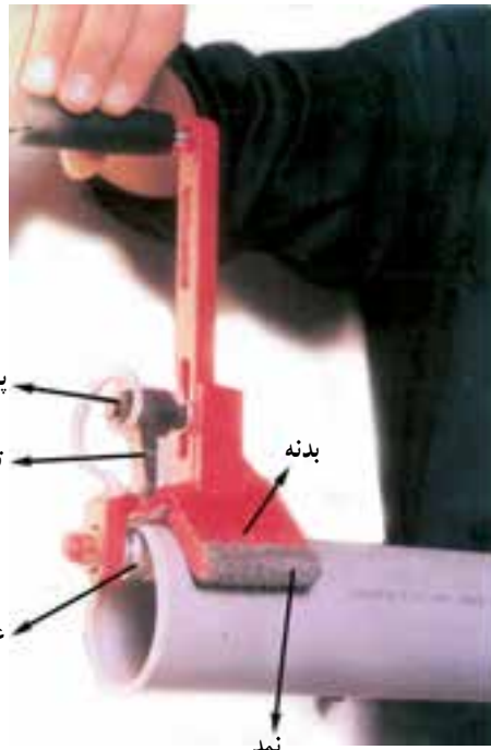
شکل ۲-۷۲ - دسته
