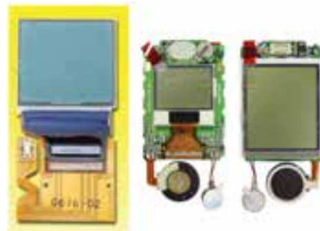
شکل ۱۹-۳۰- اجزای واحد نمایش
