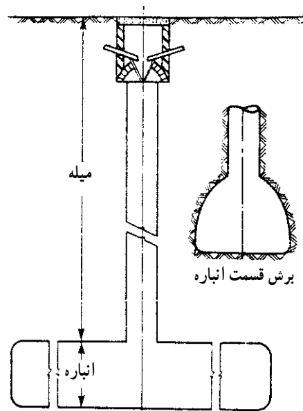
شکل ۱۱-۸- نمای کلی یک چاه فاضلاب
