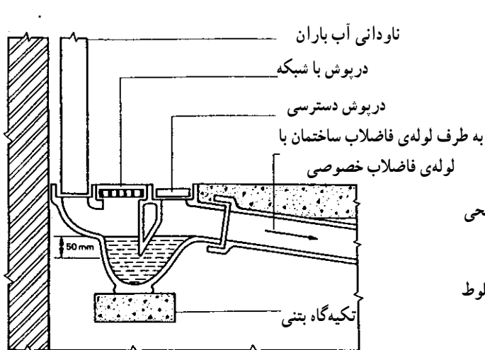
شکل ۱۱-۱۱- چگونگی دفع آب باران و آب‌های سطحی
