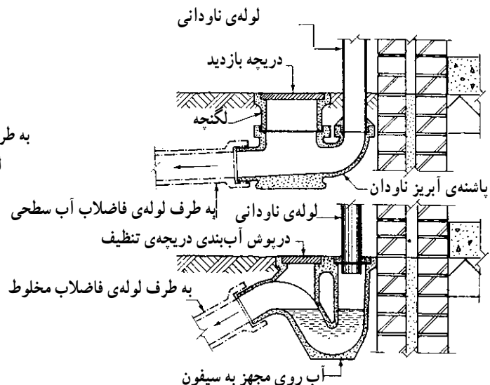
شکل ۱۱-۱۱- چگونگی دفع آب باران و آب‌های سطحی
