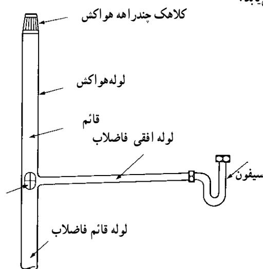
شکل ۱۱-۱-۱ اجزای یک سیستم فاضلاب
