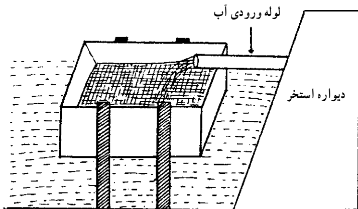
شکل ۱۵-۴- فیلتر داخل استخر برای گرفتن آبریان هرز
