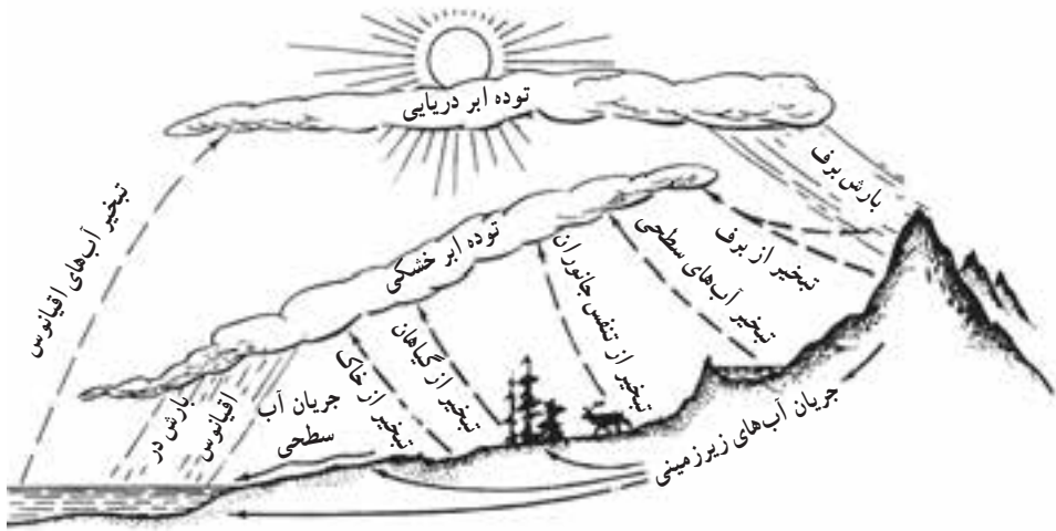
شکل ۱-۴- چرخه آب
