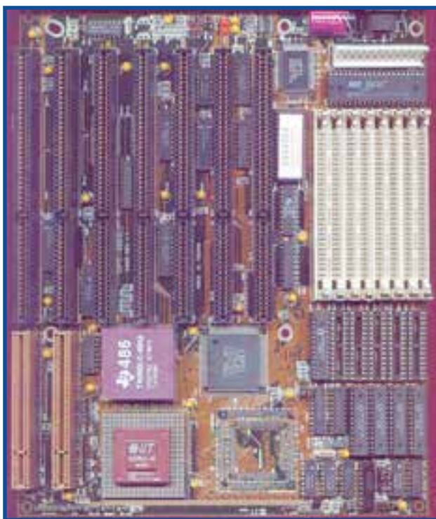
شکل ۴-۲ برد اصلی AT به همراه پردازنده ۴۸۶ و شکاف‌های SIMM
