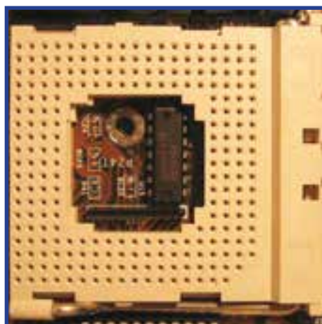
شکل ۲۲-۳ پردازنده ۴۱۰۰ DX ۴۸۶ با سرعت ۱۰۰ مگاهرتز و سوکت شماره ۳
