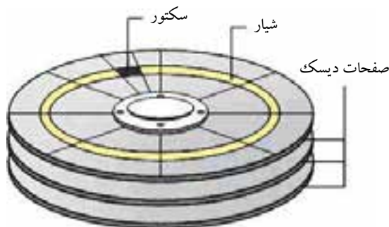
شکل ۳۲-۴ سکتور، شیار و سیلندر در صفحات مختلف دیسک سخت
