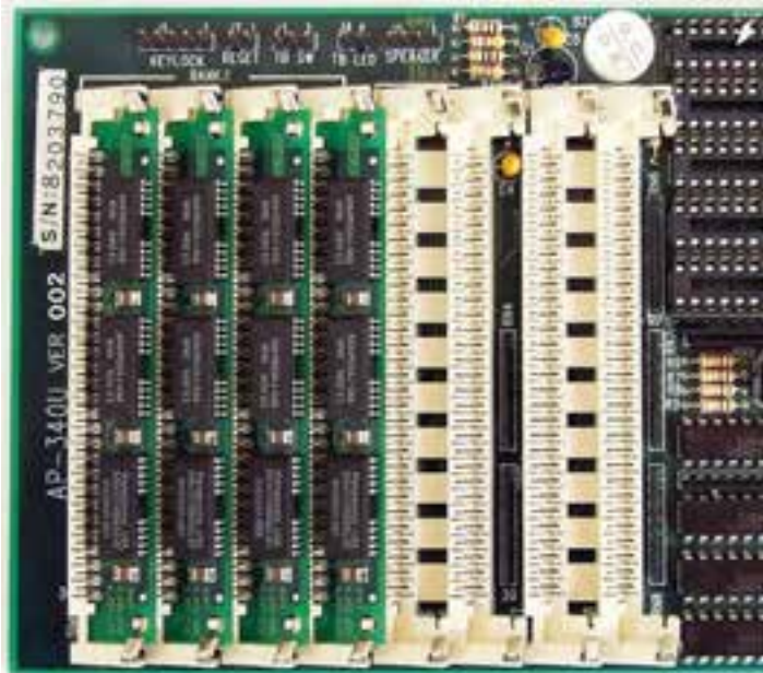
شکل ۱۰-۴ ماژول‌های SIMM که تراشه‌های حافظه در یک طرف آن قرار می‌گیرد و شکاف‌های مربوط به آن روی برد اصلی (رنگ سفید)
