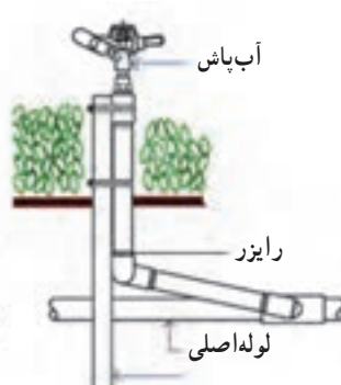
(الف) آب‌پاش نصب شده روی رایزر
