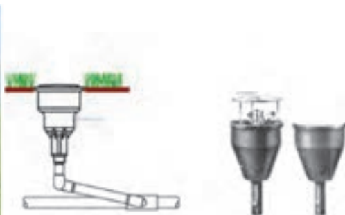
الف) ساختار آب پاش مخفی شونده ب) چگونگی نصب آب پاش
