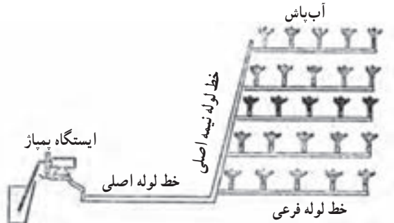
شکل ۷-۸- شبکه لوله‌ها در آبیاری بارانی
