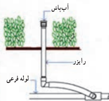
(الف) لوله فرعی زیر زمینی و رایزر
