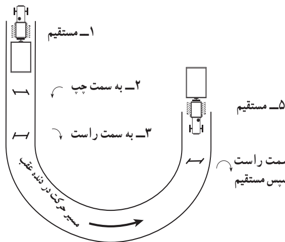
شکل ۳۴-۱ دور زدن در دنده عقب با پی نورد
