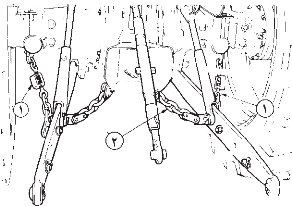
۱- زنجر خارجی ۲- زنجر مہار داخلی
