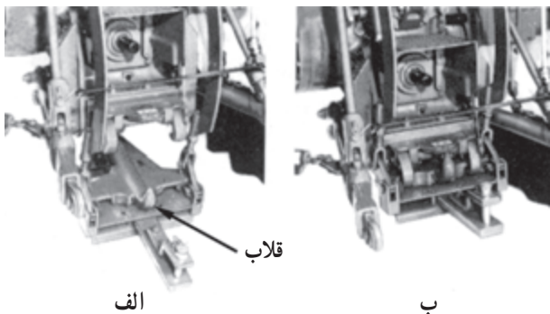
الف - مالبند هیدرولیکی در حالت باز ب - مالبند هیدرولیکی در حالت بسته شکل ۱-۵۱ - مالبند هیدرولیکی در تراکتور JD3050
