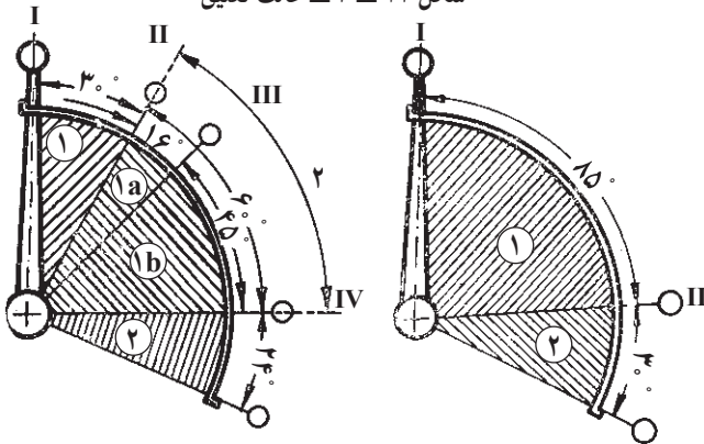
الف ب الف - اهرم انتخاب در حالت کنترل وضعیت ب - اهرم انتخاب در حالت کنترل بار ۱- وضعیت های مختلف از نظر ارتفاع ۲- تعلیق
