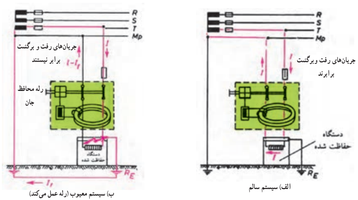
شکل ۱۱-۱۰ مدار الکتریکی کلید محافظ جان
