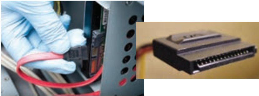
شکل ۸-۲۴ کابل برق و کابل انتقال داده‌های SATA و روش اتصال آن
