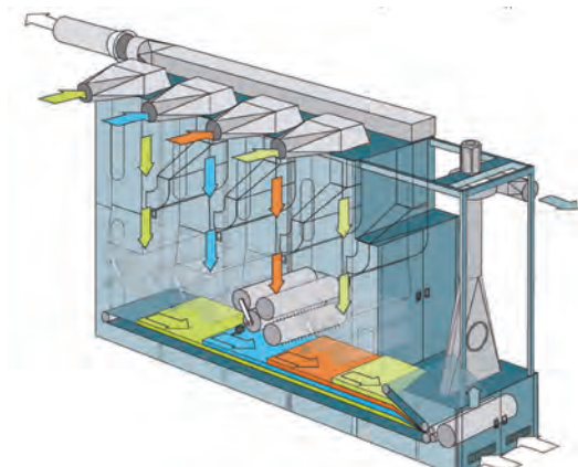
شکل ۴۷- سوپر بلندر (تغذیه با چند ورودی شوت فید)
