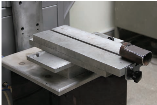
شکل ۵-۸ بستن قالب جای میز دستگاه
