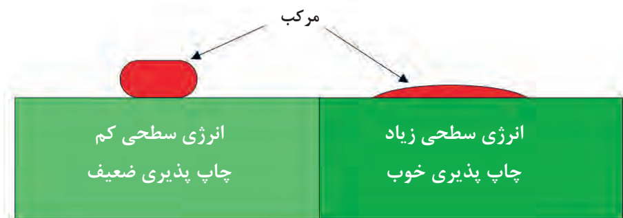
شکل ۳-۳۸ کشش سطحی در چسبندگی در مواد خیس پذیر و خیس ناپذیر
