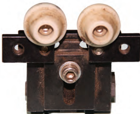
شکل ۲۵-۵ فیکسچرهای بلبرینگ دار
