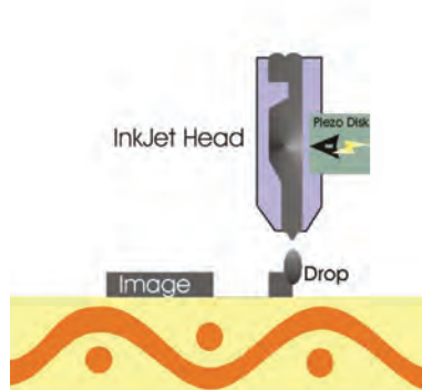
شکل ۱۴-۱ الف- نگاشت طرح روی قشر امولسیون
