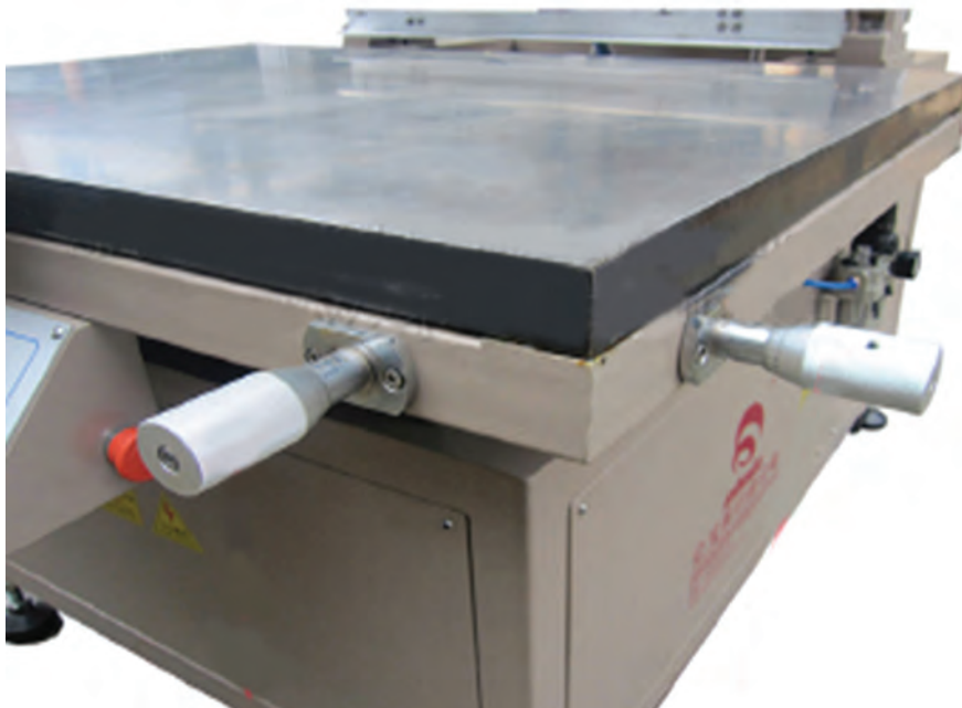
شکل ۳-۴ گونیا کردن طولی و عرضی با صفحه متحرک میز کار
