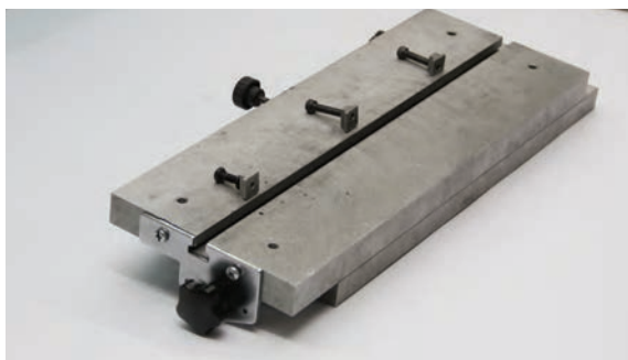
شکل ۵-۲۶ میز شیاردار- فیکسچر به همراه مهره های
