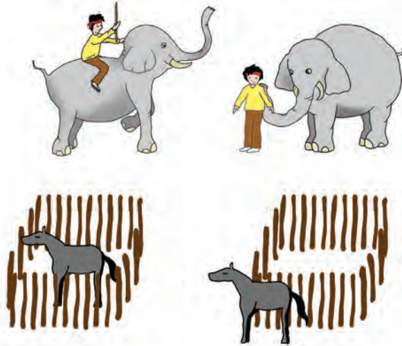
شکل ۳۱- مفهوم مکانی
