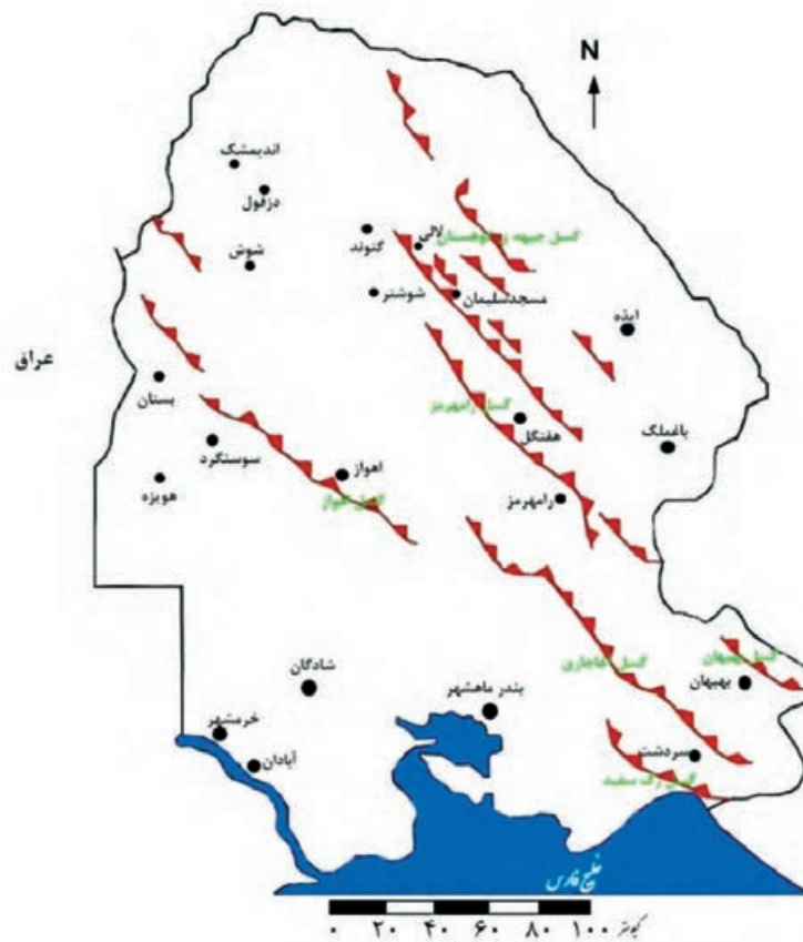
شکل ۵-۱- گسل‌های استان
