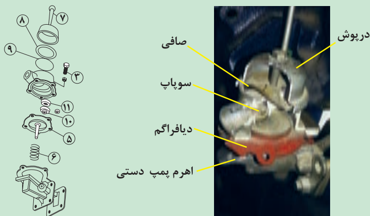
شکل ۳۷. شکل شماتیک و نمای برش خورده پمپ مقدماتی تراکتور MF285
